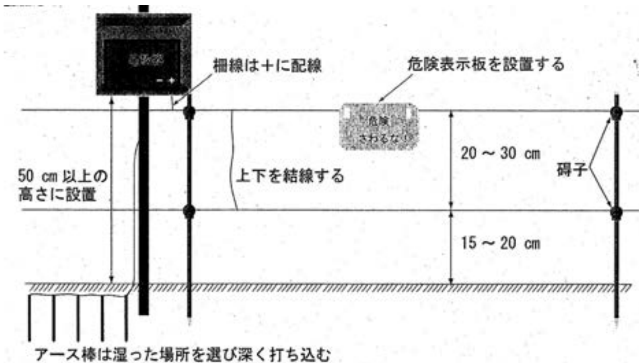
電気柵（電線型で2段）の正面図
