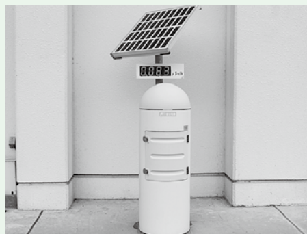
リアルタイム線量測定システム
