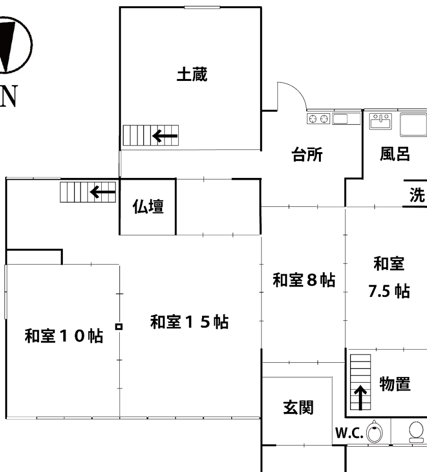
1階間取り
